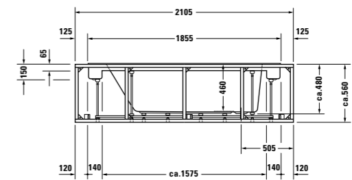
# 700125 00 0 00 0000, 2000 x 1000 mm + # 790831 00 0 00 0000, Auffaltbares Ruhedeck. Relaxations deck. Copertura imbottita pieghevole. Banquette de relaxation. Inklapbaar zonedek. Tumbona plegable + # 790153 00 0 00 0000, Schienensystem. Rail-mount system. Sistema a binari. Système de rails. Railmodule. Sistema de perfiles Einbauversion. Built-in. Versione da incasso. Version à encastrer. Inbouwversie. Versión empotrada
